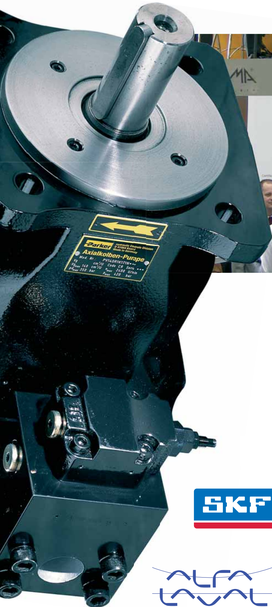
Axiální pístové čerpadlo PV ■ Axial piston pump PV
